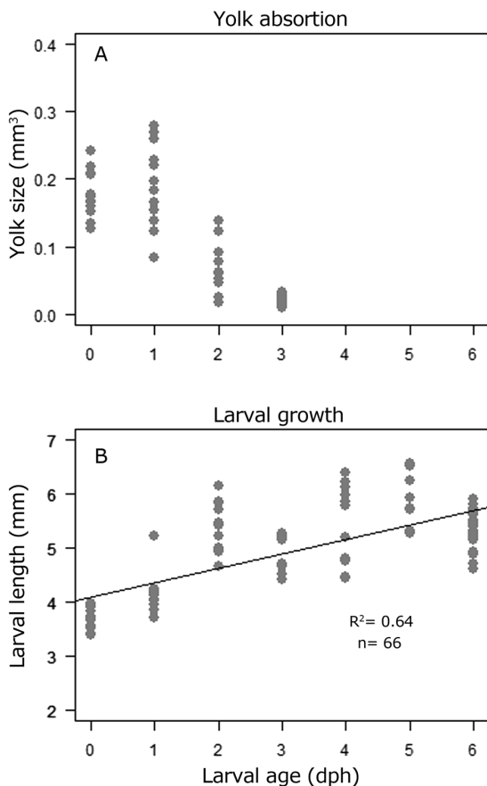
Figure 3. Patagonian sprat yolk sac absorption (A) and larval growth (B), under laboratory conditions / Absorción del saco vitelino (A) y crecimiento de las larvas (B) de sardina austral bajo condiciones de laboratorio
